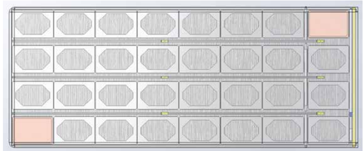
Beispiel einer Filialeinteilung ohne Radkästen auf Basis Tiefrahmenfahrstell
